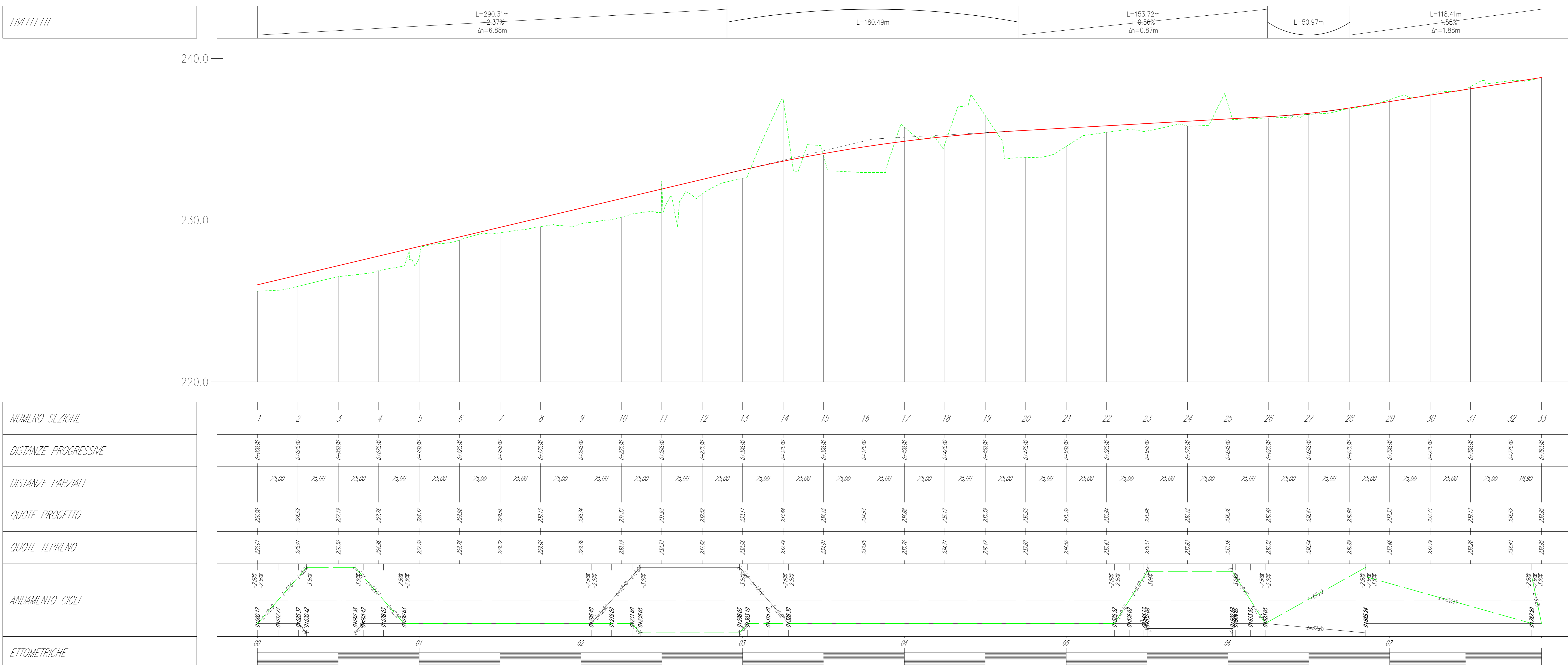
PROFILO LONGITUDINALE NUOVO TRONCO TRATTO 4 scala 1:1000/100
